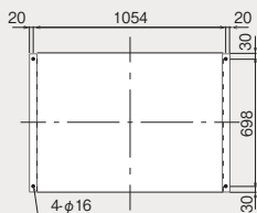
B矢視 基礎図
