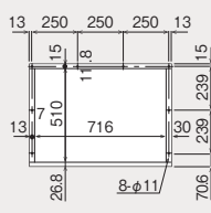
A矢視 吸込ダクト接続口
