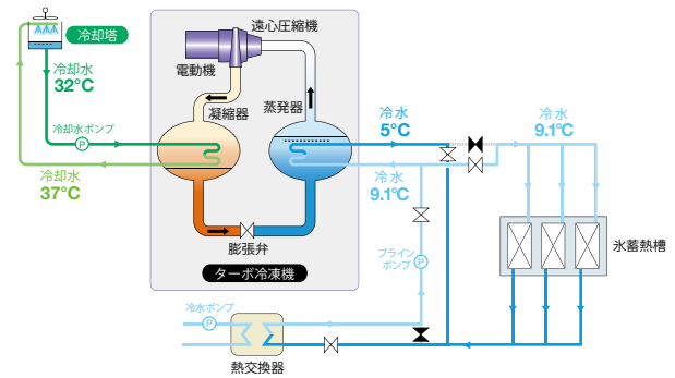
システムフロー図 【追掛運転（昼）】
