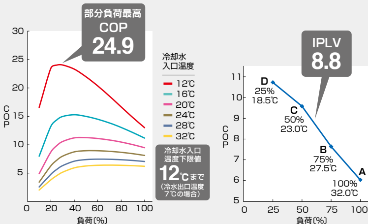
部分負荷特性 (JHT-Y245I)
