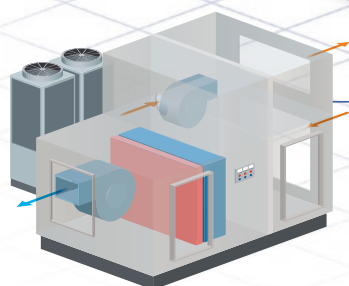
⑬ 冷媒再熱型調湿外気処理機 LXC-H(EHP) LXCP-RF(EHP)
