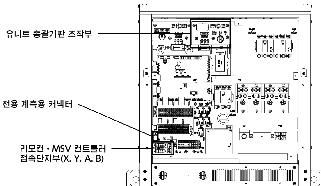
<전원박스>
