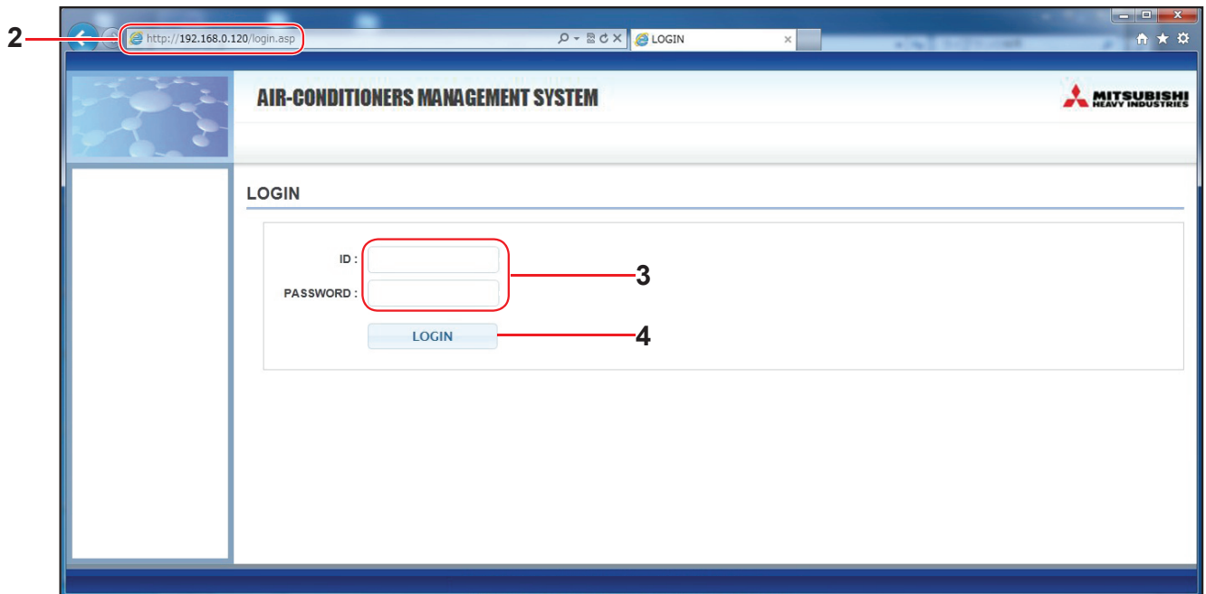
LOGIN-scherm
