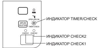
ИНДИКАТОР CHECK2 ИНДИКАТОР TIMER/CHECK
