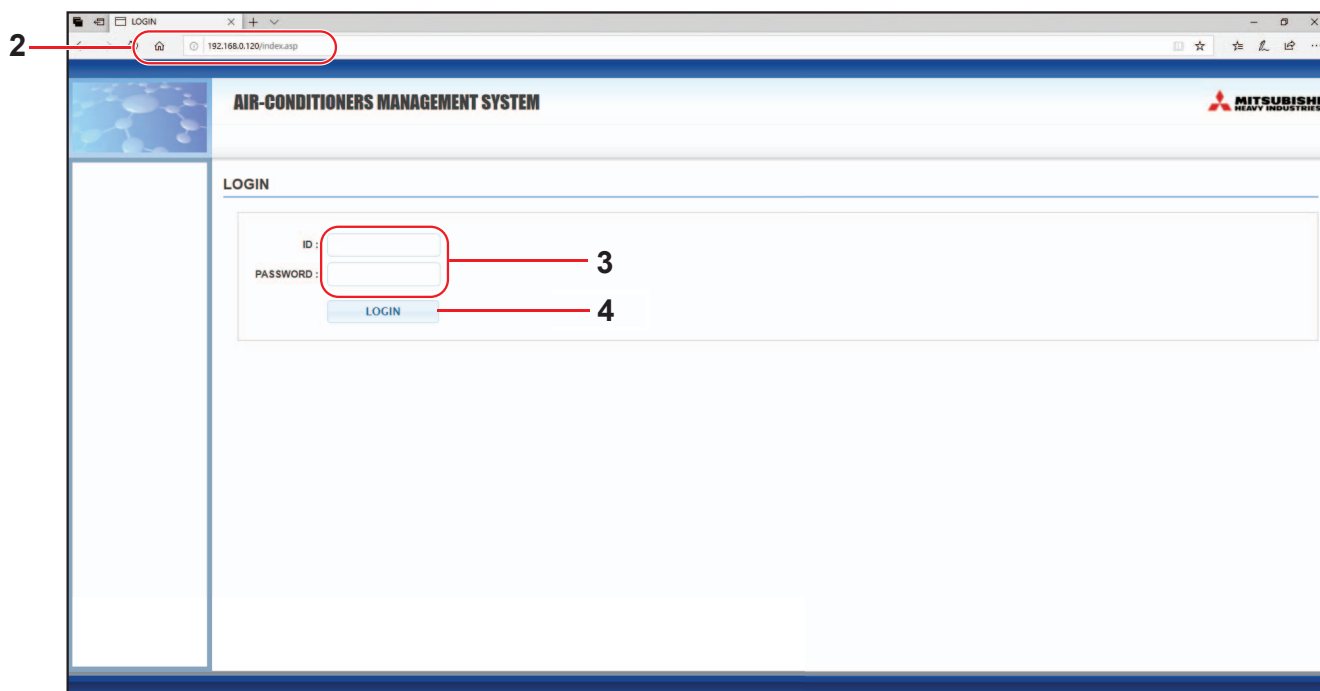
Pantalla LOGIN
