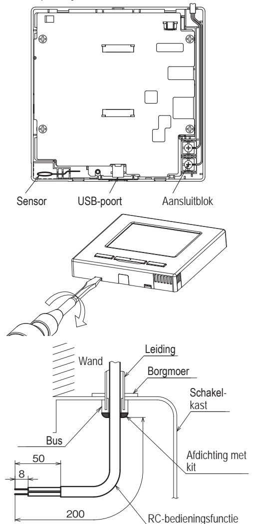
Printplaatzijde (achteraanzicht)
