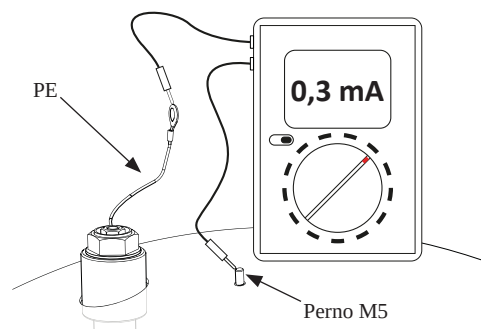
Misurazione dell'intensità della corrente continua di protezione
