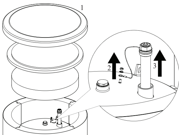
Remplacement de l'anode protectrice en magnésium
