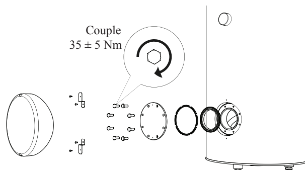
Installation du couvercle d'ouverture et d'inspection (ordre de montage).
