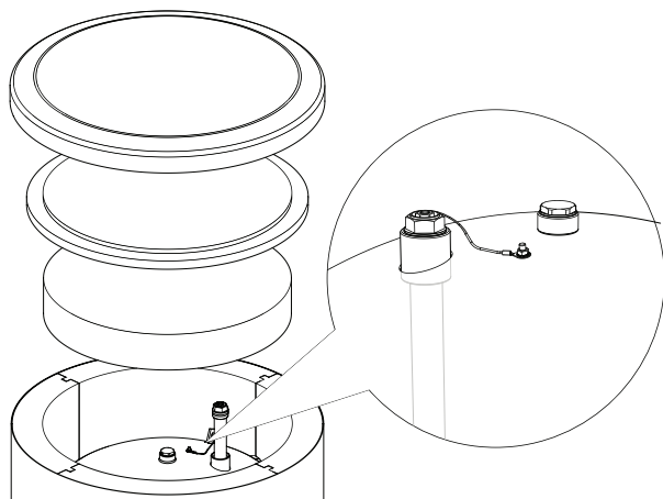
Anode protectrice en magnésium isolée
