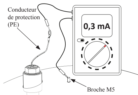
Mesure de l'intensité du courant continu de protection
