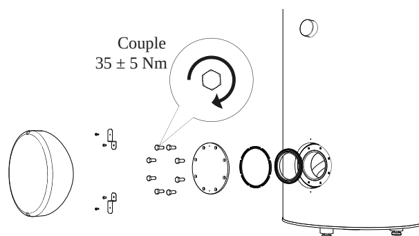
Installation du couvercle d'ouverture et d'inspection (ordre de montage).
