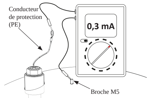
Mesure de l'intensité du courant continu de protection
