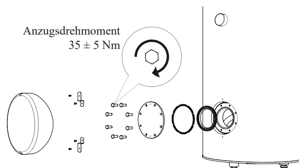
Die Abdeckung der Installationsöffnung anbringen (Montagereihenfolge).
