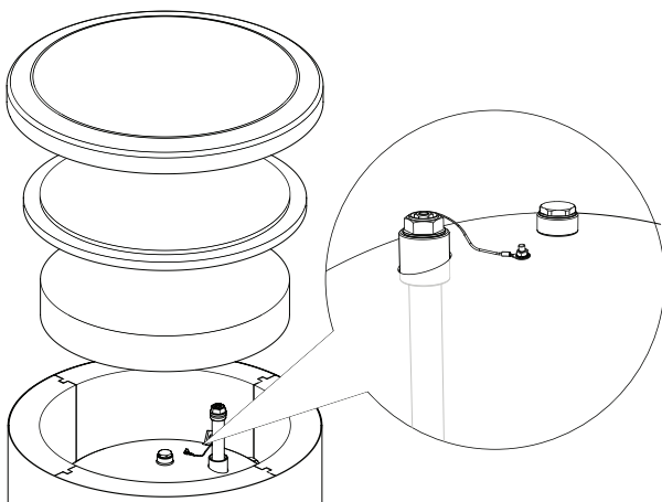
Isolierte Magnesium-Opferanode
