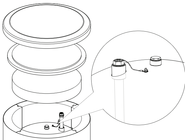
Anodo di protezione in magnesio isolato
