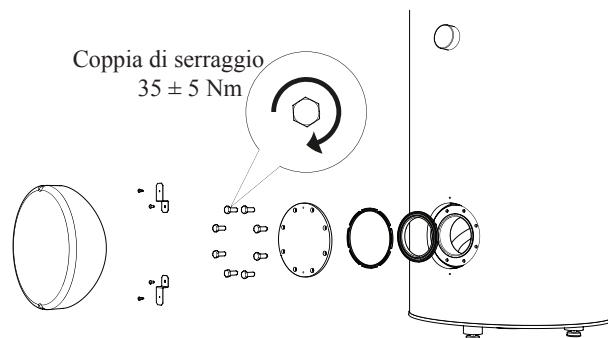
Installazione del coperchio dell'apertura di ispezione (sequenza di montaggio).
