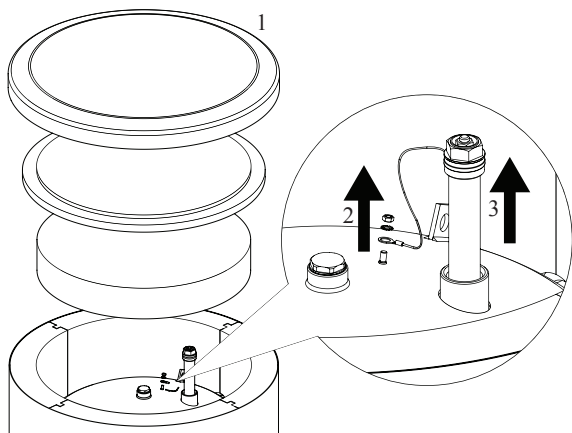
Sostituzione dell'anodo di protezione in magnesio
