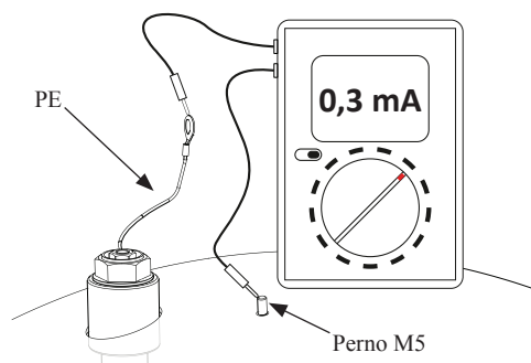
Misurazione dell'intensità della corrente continua di protezione
