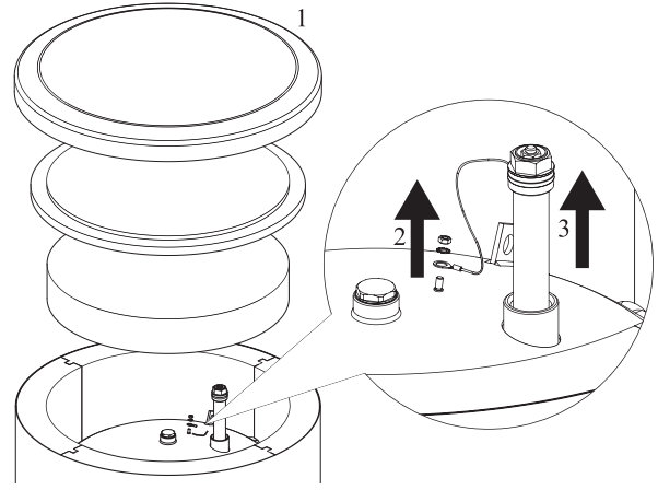
Koruyucu magnezyum anotun değiştirilmesi
