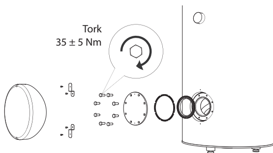
Muayene açma kapağının yerleştirilmesi (takma sırası)
