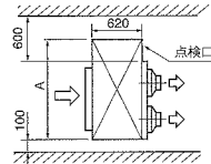
(室内機) 据付スペース
