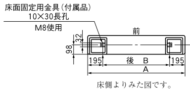
床面固定金具用ボルト位置
