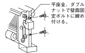
壁面固定の場合
