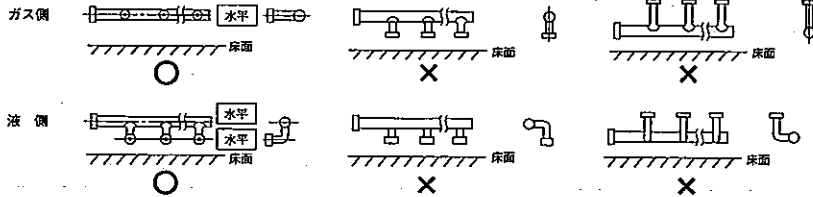
ユニット配管仕様 配管材質は、リン酸銅鍍目黒鋼管 (C12207, JIS H3300)
