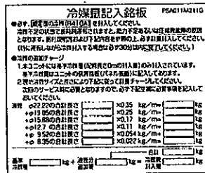
冷媒量記入銘板
