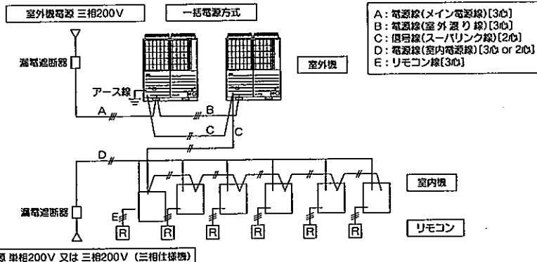
室内機電源 単相200V 又は 三相200V (三相仕様機)
