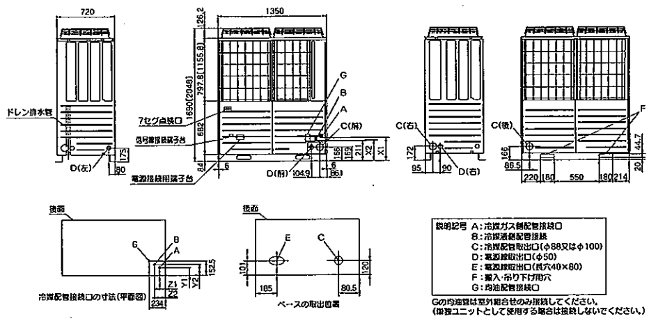
6) 配管接続位置と配管取出方向
