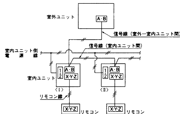
〔室外・室内ユニット接続要領〕
