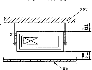
正面図 (単位: mm)
