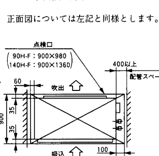
平面図 (単位: mm)
