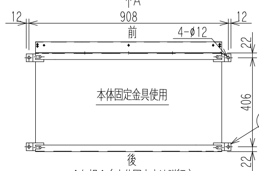
A矢視1 (本体固定方法詳細)
