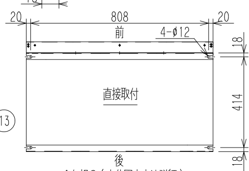
A矢視2 (本体固定方法詳細)
