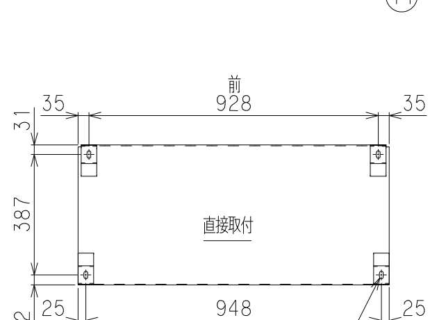
A矢視 (本体固定方法詳細)
