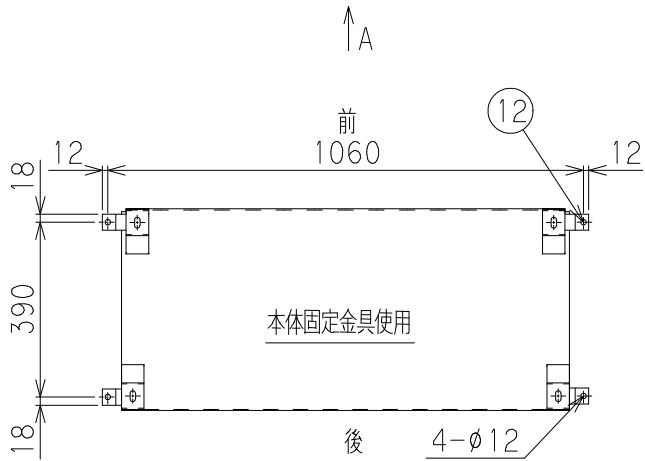
A矢視 (本体固定方法詳細)
