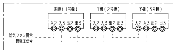
※1 接続図
