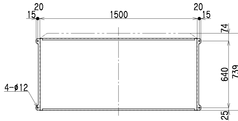
A矢視 基礎図
