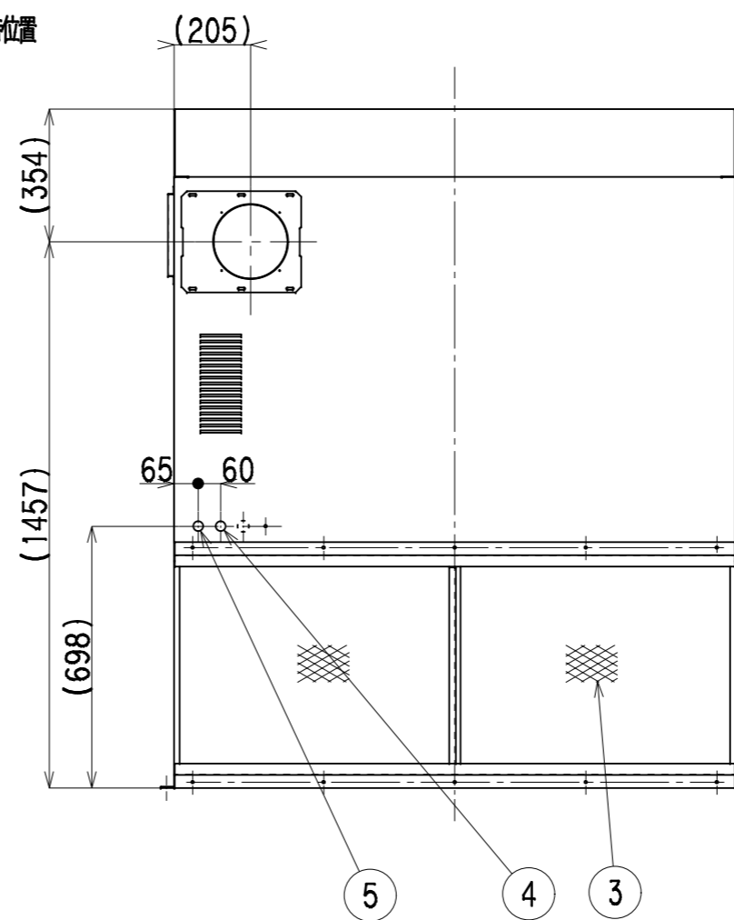
A矢視 基礎図
