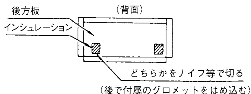
背面方向取出し
