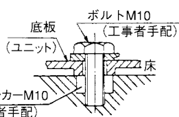
コンクリートの 床に固定
