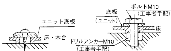
木の床又は 木台に固定
