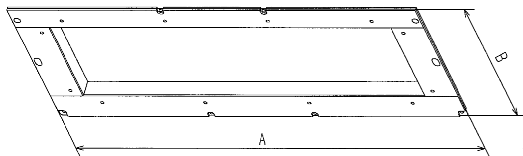
ダクトジョイント 1個
