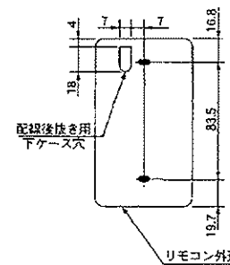
リモコン取付寸法
