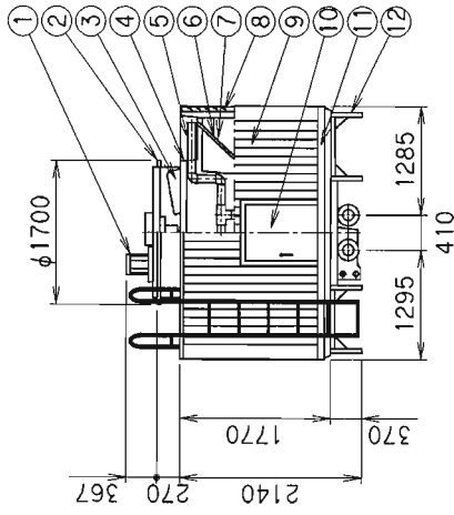
配管通り詳細図
