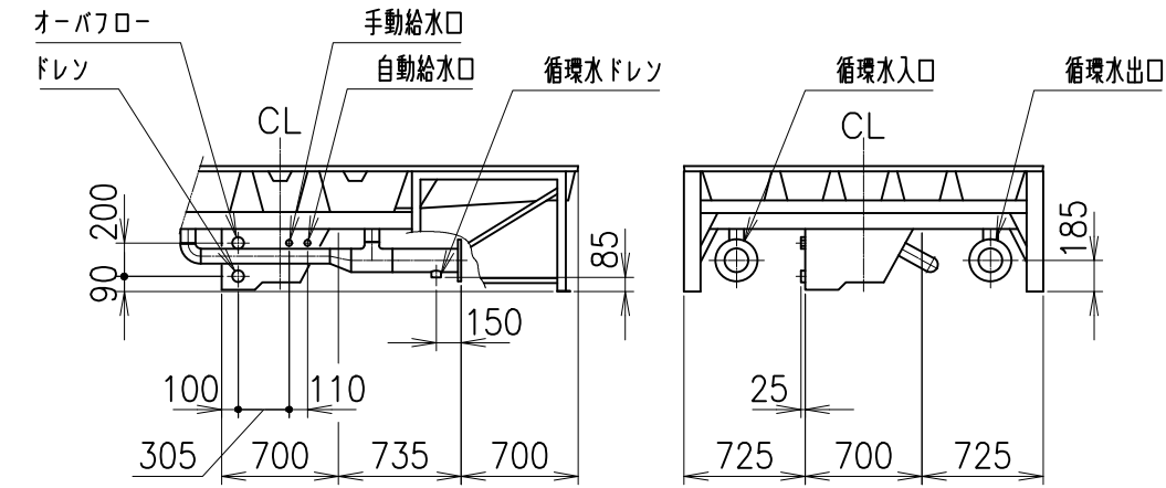
配管廻り詳細図 (S=1:50)
