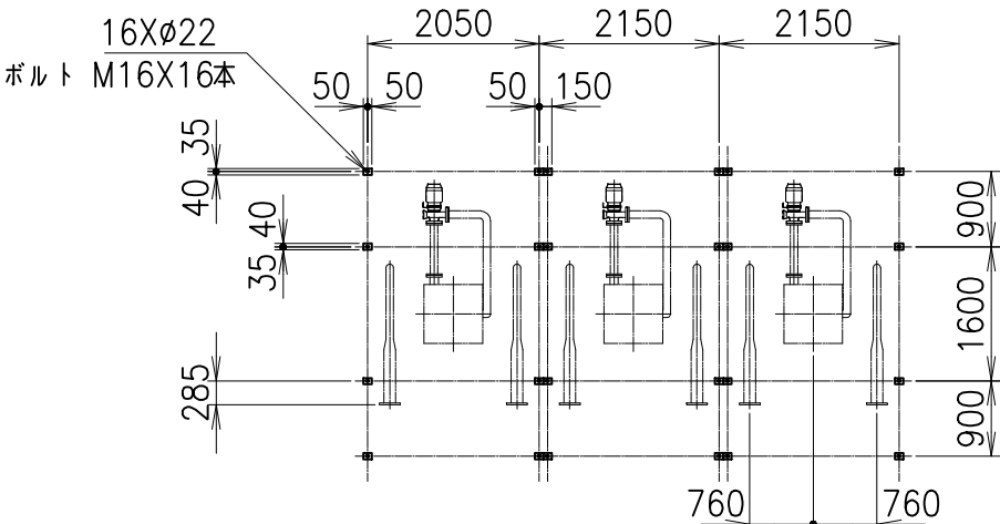
脚プレートボルト穴位置図
