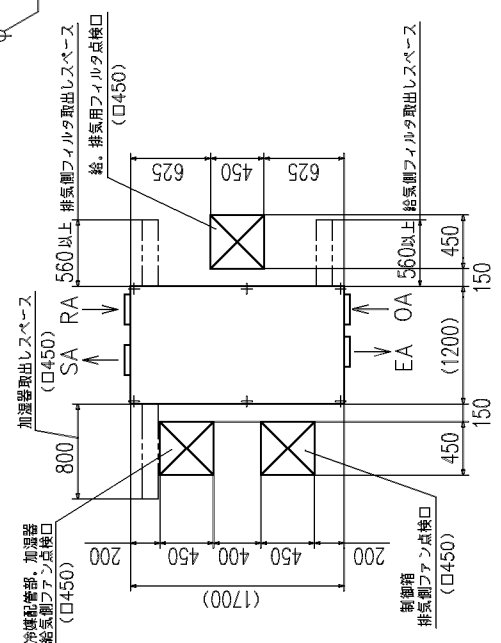
サービススペース (ユニット上面より見た配置図)
