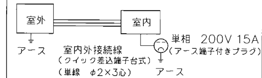
配線接続図
