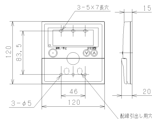
リモコンスイッチ寸法図
