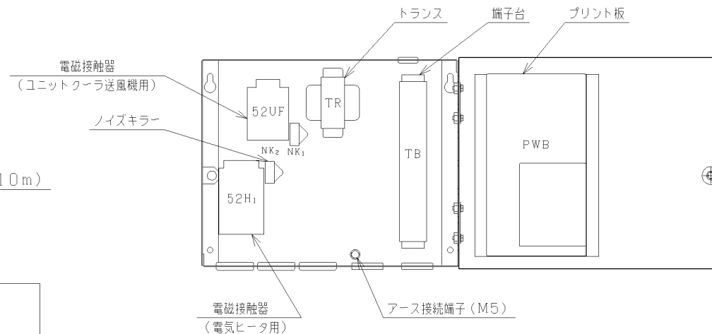
機器配置図
