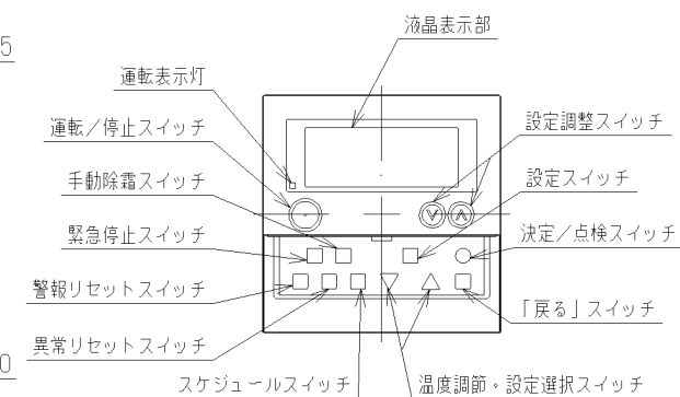
機器配置図
