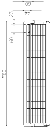
外形図(室内ユニット)
