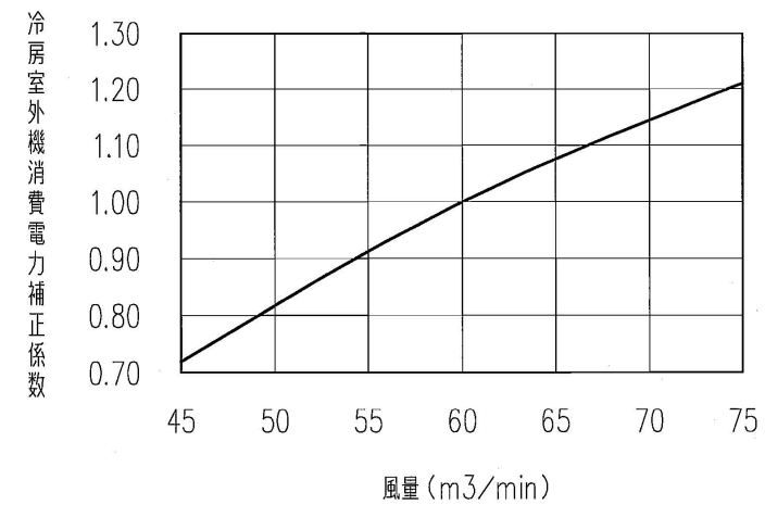
高頭熱PAC 140 冷房
