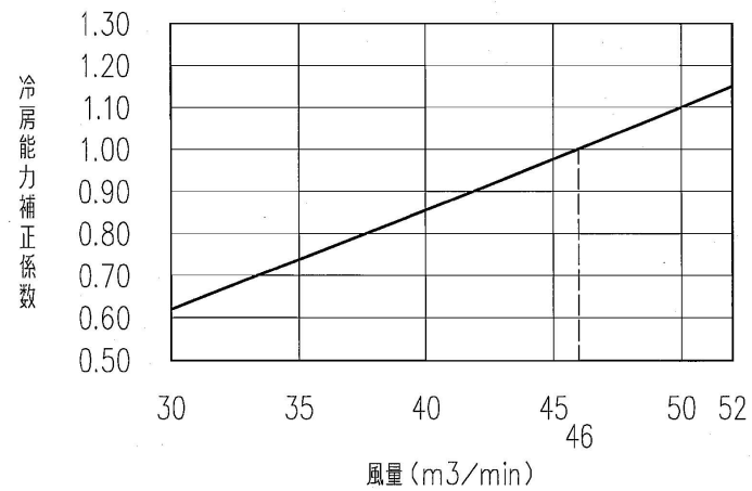
高頭熱PAC 140 冷房
