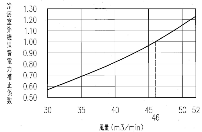
高頭熱PAC 80 冷房
