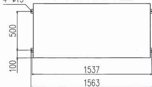
Y-Y (アンカボルト位置)
