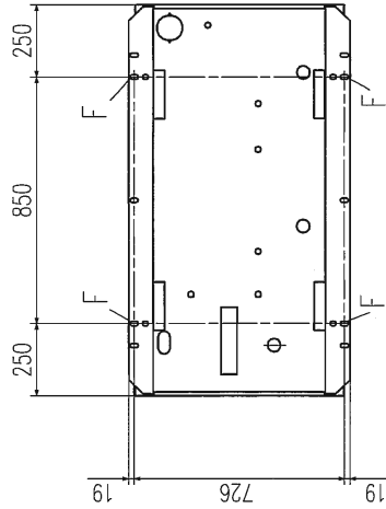
アンカーボルト用穴寸法
