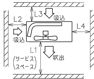
据付最小スペース
