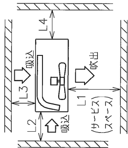
据付最小スペース
