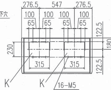
Z-Z (送風機室天井詳細)
