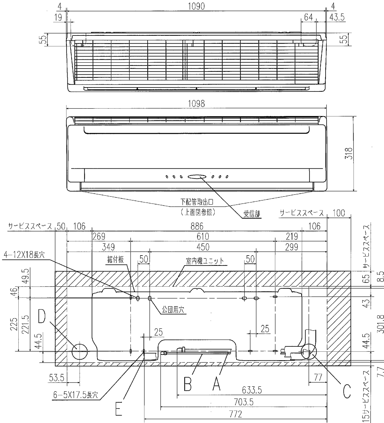
正面から見た据付け位置図及び据付けスペース
