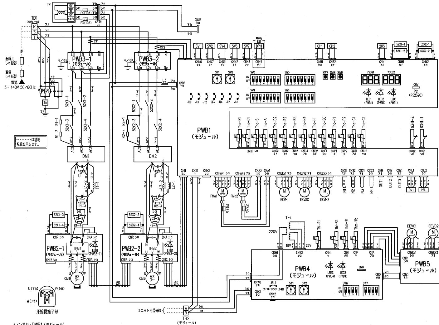
メイン基板: PWB1 (モジュール)
