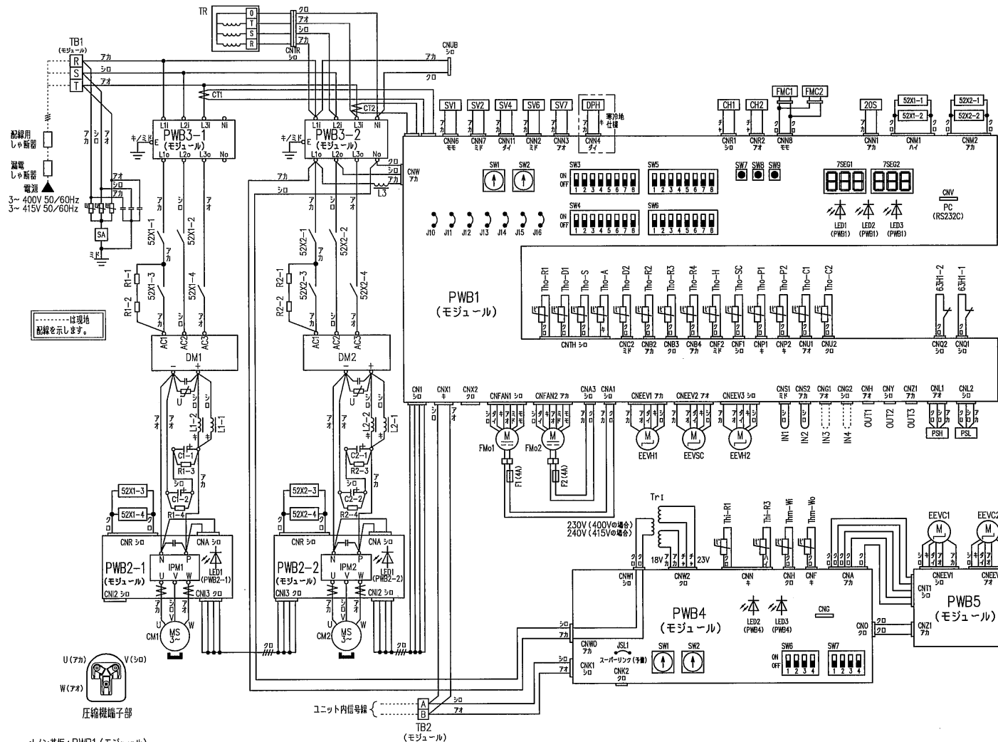
メイン基板: PWB1 (モジュール)
