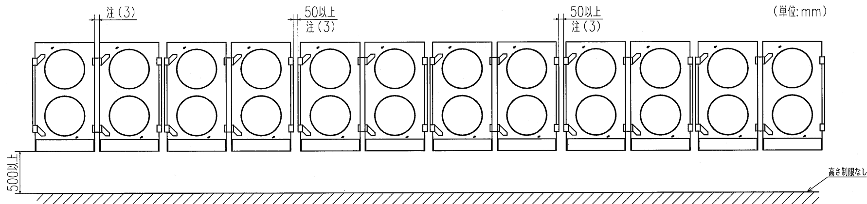
据付スペース (集合設置の場合)
