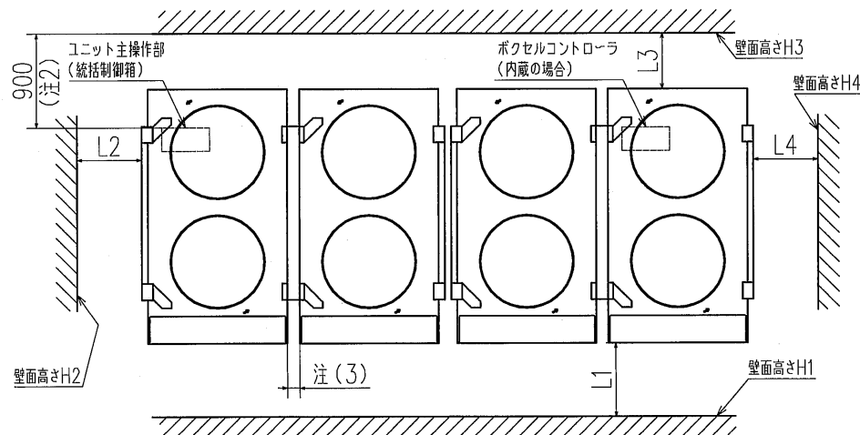
据付スペース (1ユニットの場合)
