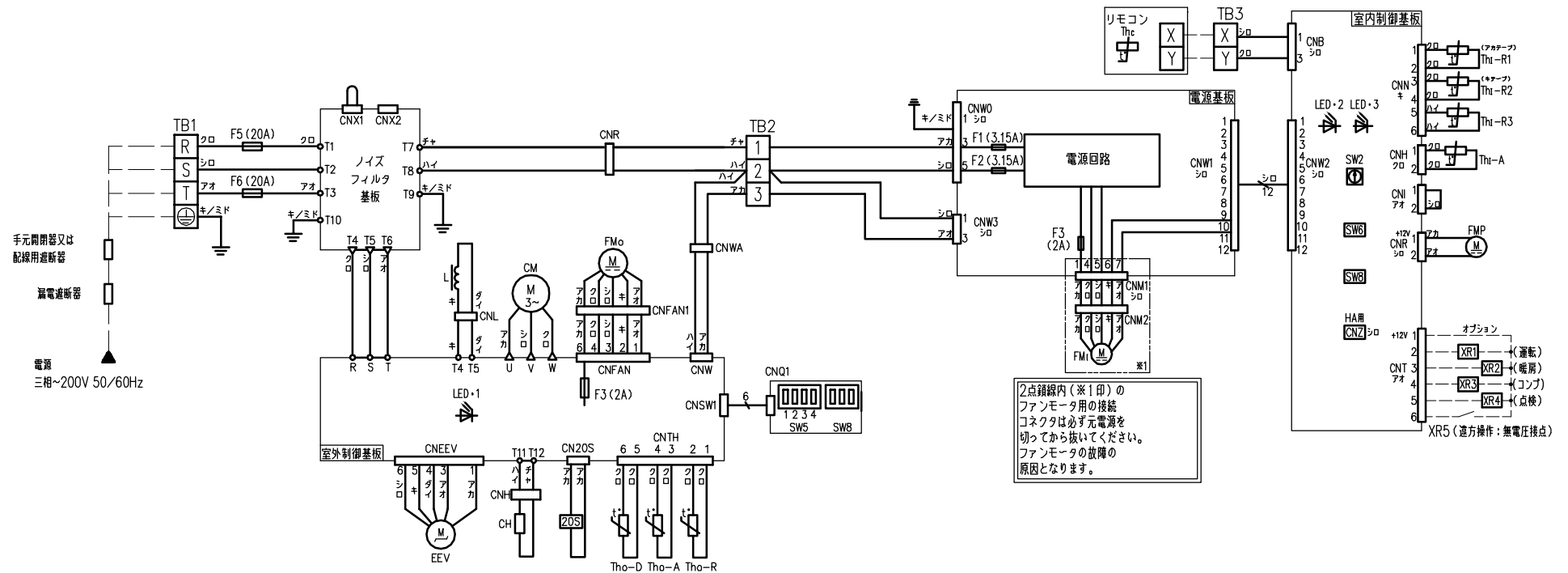
室外制御基板・記号
