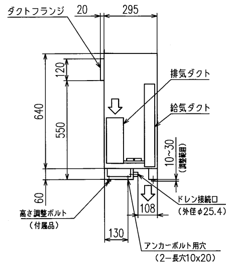
ドレン接続要領 (A-A)
