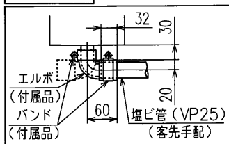
ドレン接続要領 (A-A)
