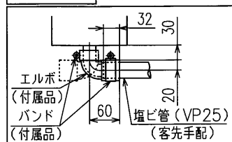
ドレン接続要領 (A-A)
