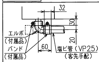
ドレン接続要領 (A-A)
