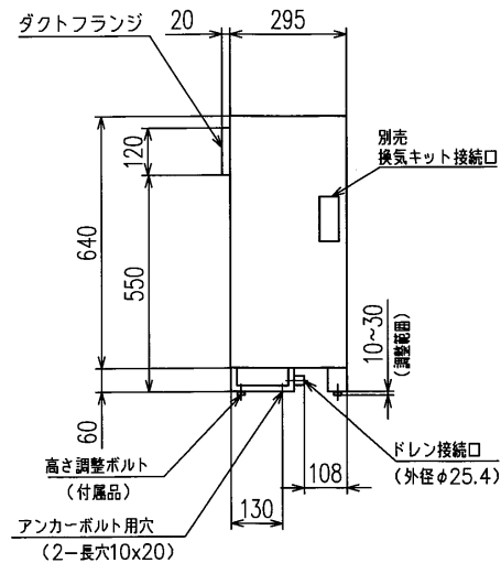
ドレン接続要領 (A-A)
