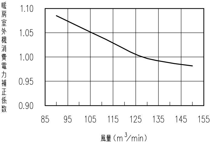
標準機 450 暖房
