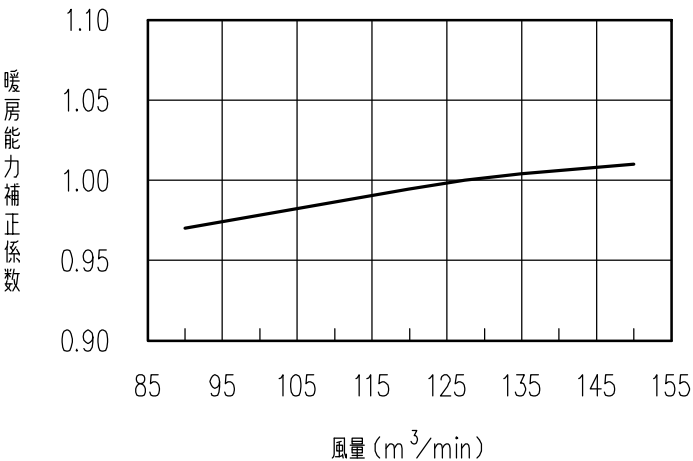
標準機 450 暖房
