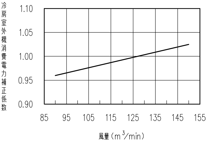
標準機 450 冷房
