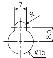
A部詳細図 (取付穴)
